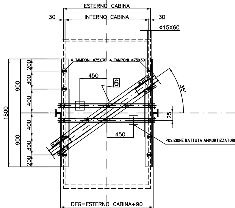
fissaggio inferiore cabina
