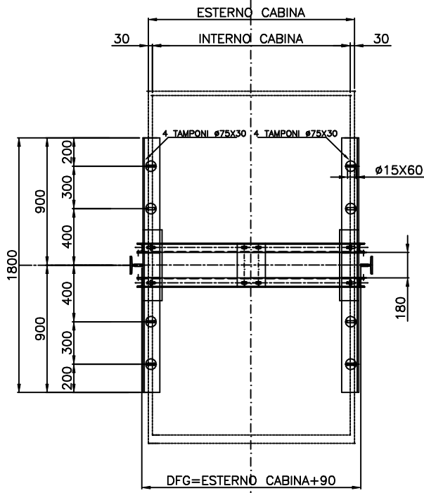
fissaggio inferiore cabina
